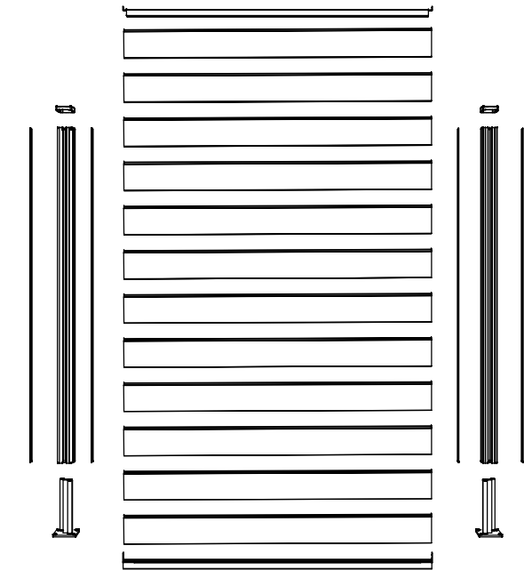
Съставни части на типов модул от системата
